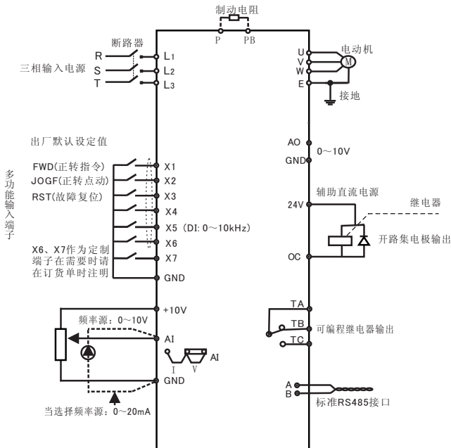
图3-3 基本接线示意图(1)
