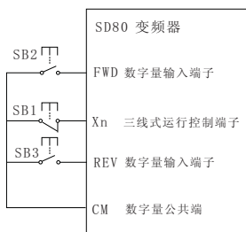
图6-6 三线式运转模式1示意图
