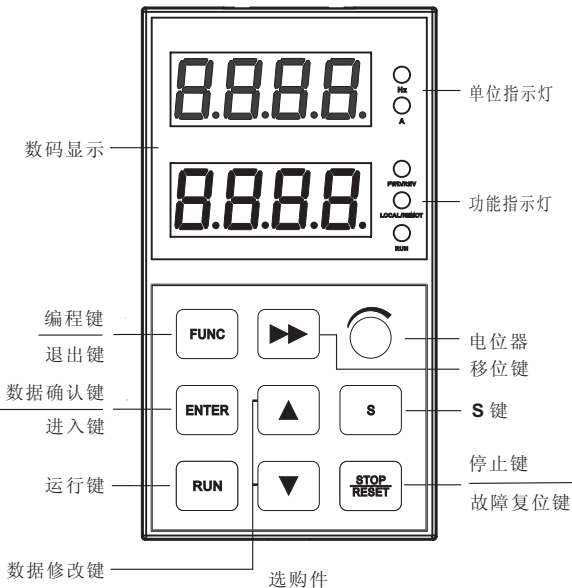
图4-2 SD80 KBB键盘示意图
