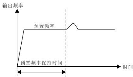
图6-19 PID预置频率示意图
