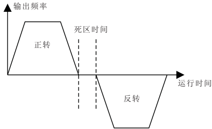
图6-15 正反转死区时间示意图
