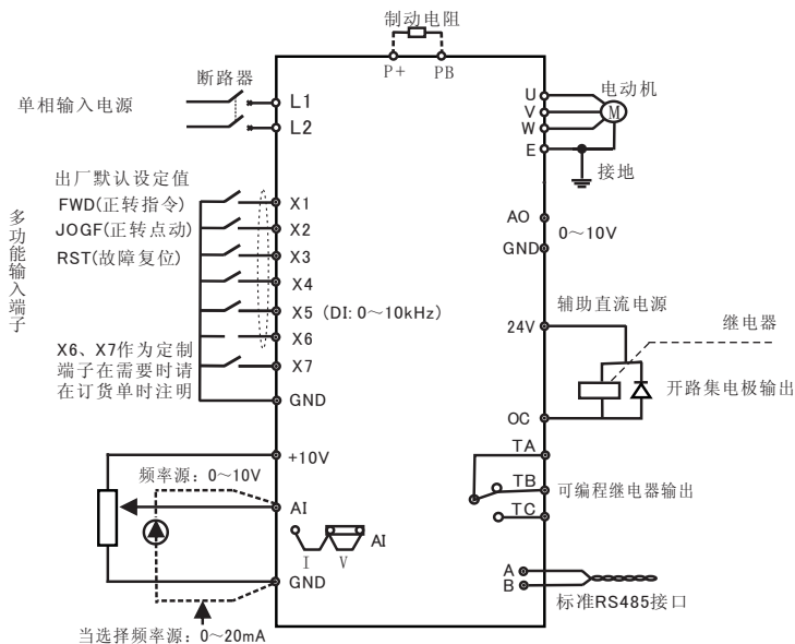
图3-4 基本接线示意图(2)
