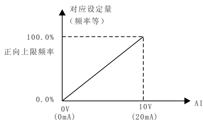
图6-8 模拟给定作为主频率源给定与输出频率的关系图
