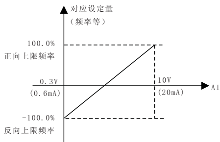
图6-10 操作杆方式：模拟给定与设定量的对应关系
