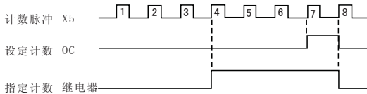
图6-22 设定计数值给定和指定计数值给定示意图
