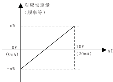
图6-9 模拟给定作为辅助频率源对主频率源进行微调
