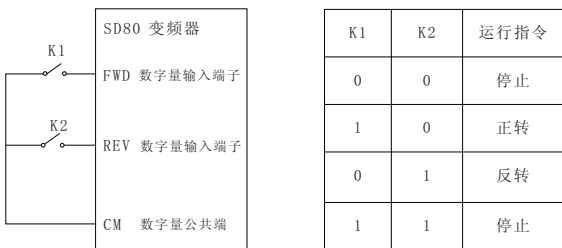
图6-4 两线式运转模式1示意图
