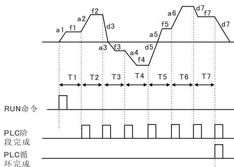
图6-24 单次运行结束停机
