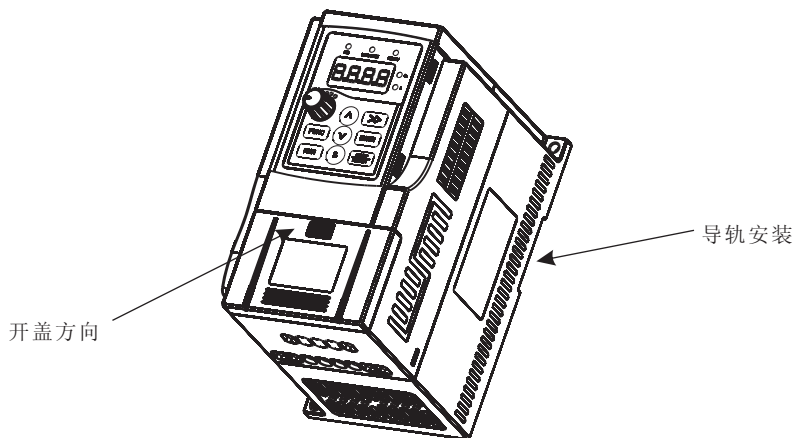
图3-2 塑胶外壳下盖板拆卸图
