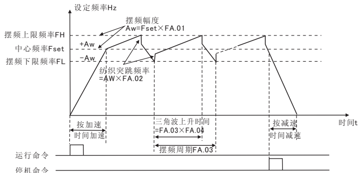
图6-21 摆频示意图
