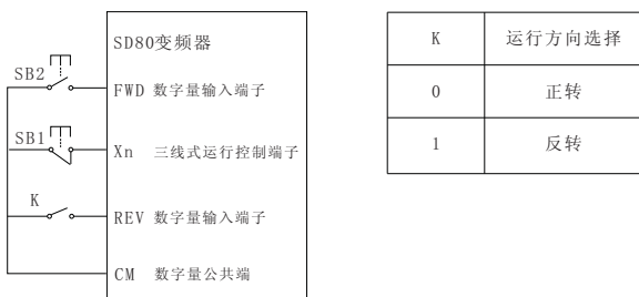
图6-7 三线式运转模式2示意图
