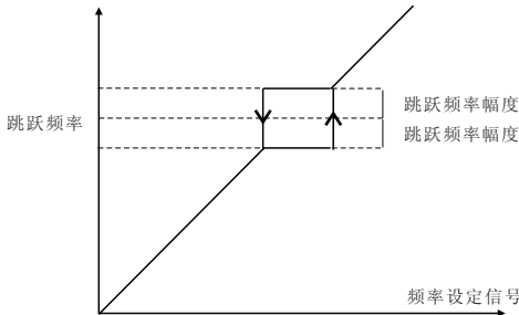
图6-14 跳跃频率示意图
