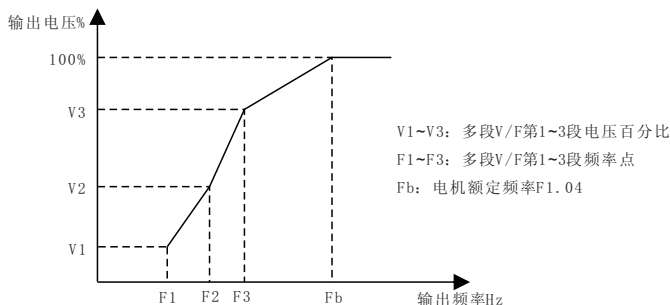
图6-2 多点V/F曲线设定示意图
