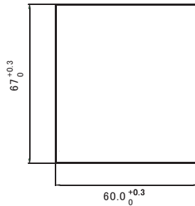
图2-6 KBC 操作面板安装开孔尺寸图
