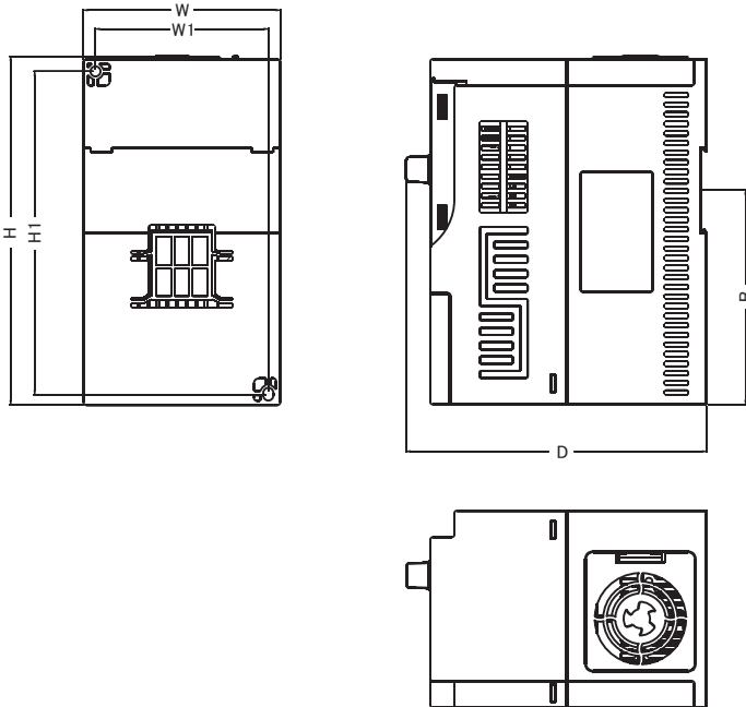
图2-3 变频器外形尺寸及安装尺寸
