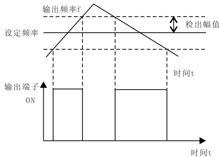
图6-17 频率到达检出幅值示意图
