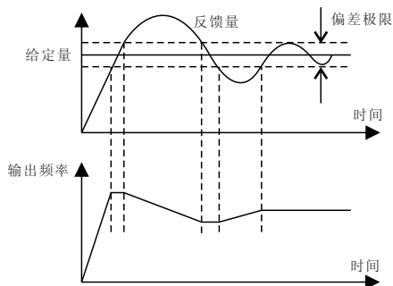
图6-18 偏差极限与输出频率的对应关系
