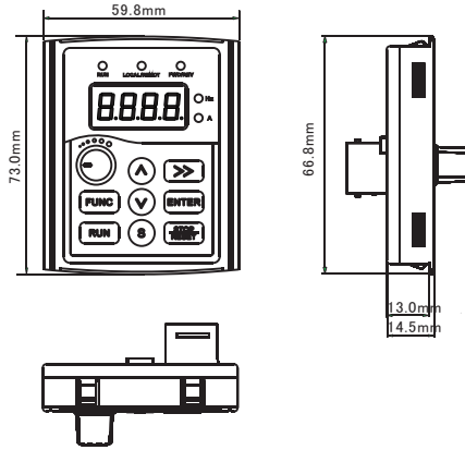
图2-5 KBC 操作面板结构尺寸图
