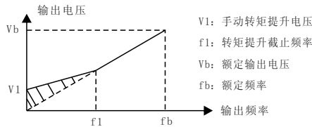
图6-3 手动转矩提升示意图
