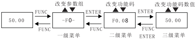
图4-3 三级菜单操作流程图
