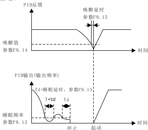
图6-20 PID睡眠唤醒示意图
