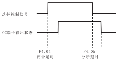
图6-11 OC输出闭合、分断延时示意图
