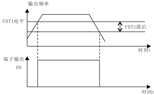
图6-16 频率水平检测示意图
