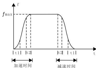
图6-13 S曲线加减速示意图
