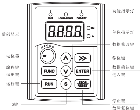
图4-1 SD80 KBC键盘示意图
