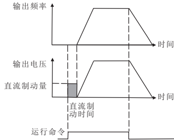
图6-12 直流制动启动方式示意图
