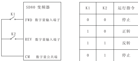
图6-5 两线式运转模式2示意图
