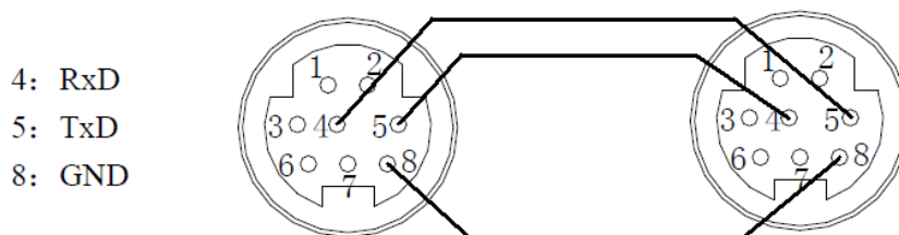
Mini Din 8 芯插座（孔）
