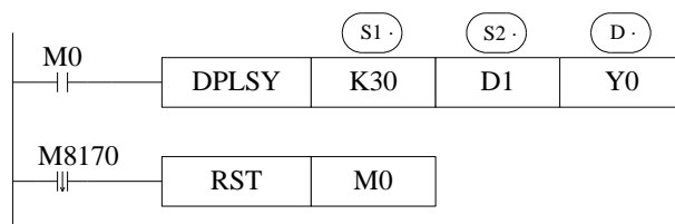
《32 位指令形式》
