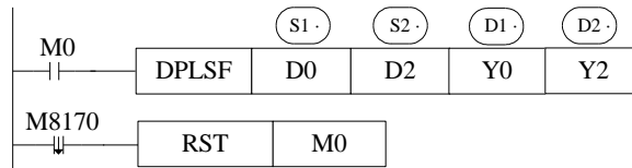
《32 位指令形式》
