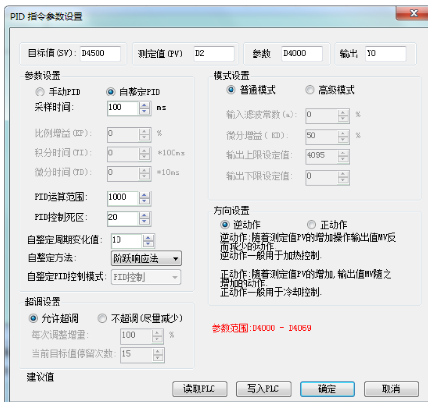
图 1 PID 自整定允许超调参数设定
