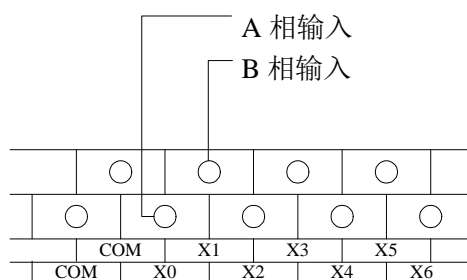
AB 相模式（计数器 HSC0）
