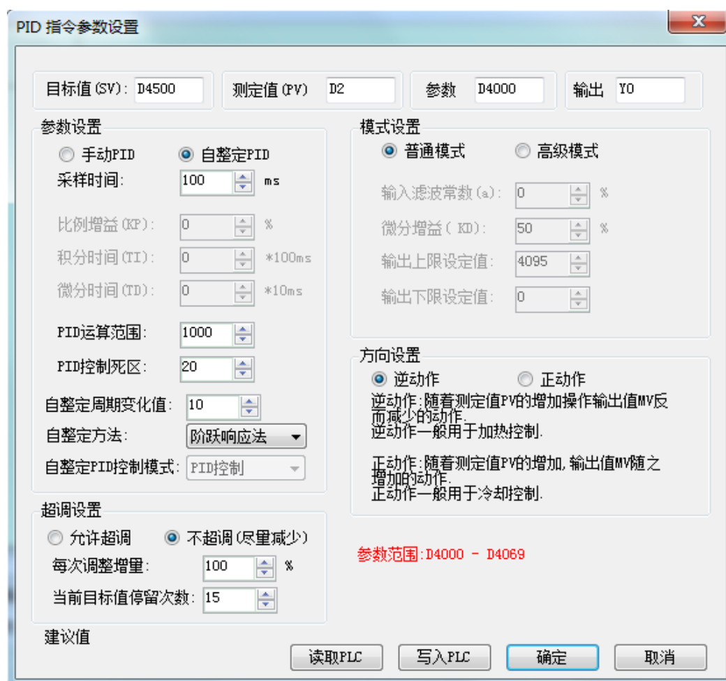
图 3 PID 自整定不允许超调参数设定
