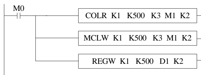
XD/XL 系列 (√)
