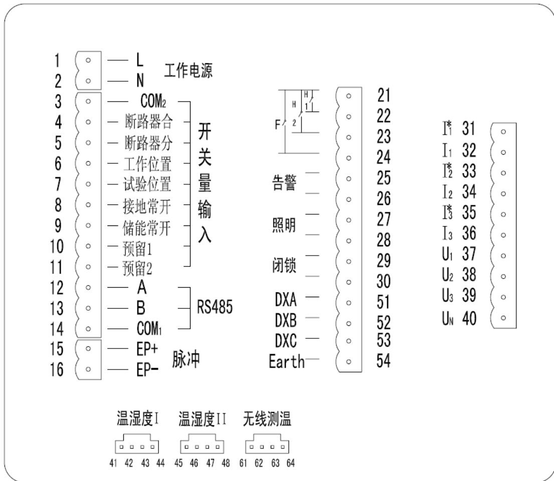
图 1.10 ASD200/300/310/320 背面端子图
