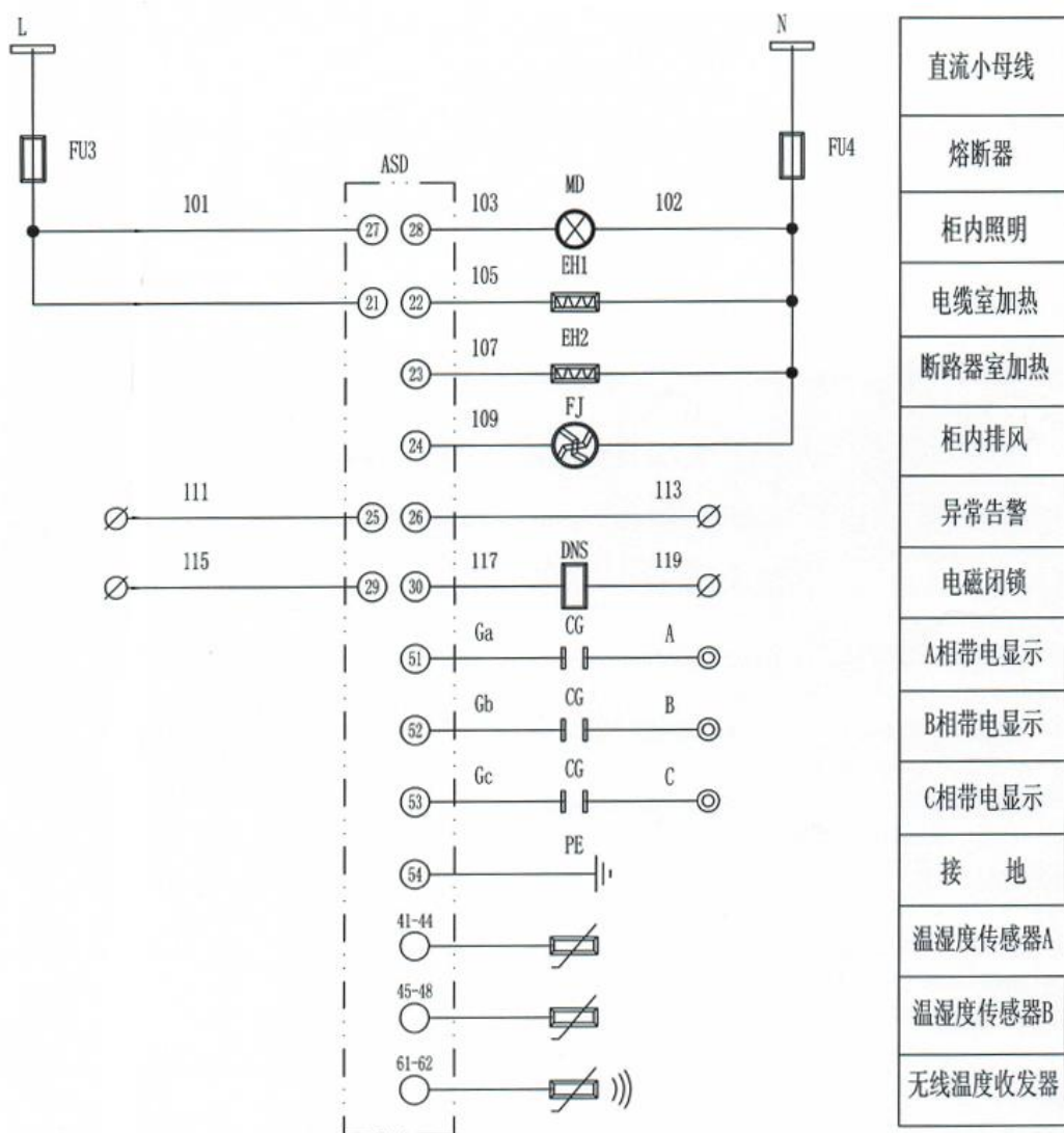
图 1.12 ASD 开关量输出、高压带电显示回路及传感器典型接线图
