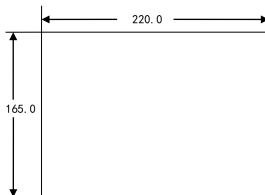
图 1.4 ASD100、ASD100G 开孔尺寸图 图 1.5 ASD200、ASD300、ASD310、ASD320 开孔尺寸
