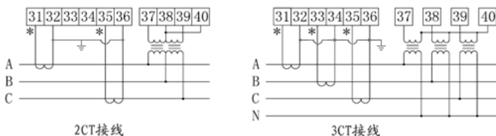
图 2.3 接线方式
