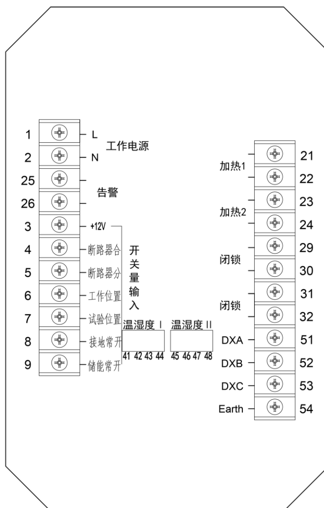
图 1.9 ASD100G 背面端子图
