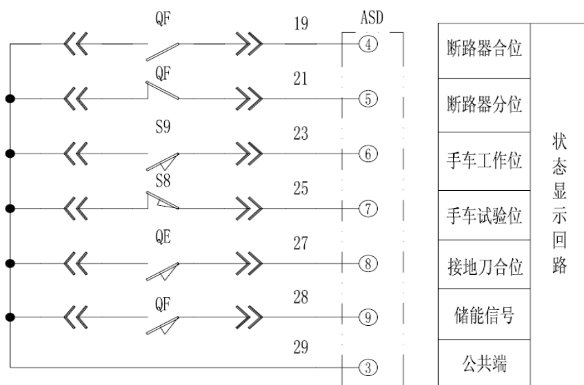
图 1.11 ASD 开关量输入回路典型接线图
